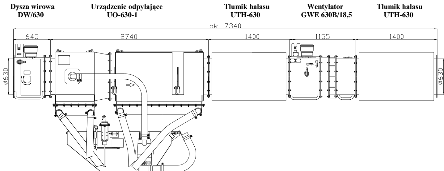
Przykład współpracy Urządzenia Odpylającego UO-630-1 z Dyszą Wirową DW/630, wentylatorem GWE 630B/18,5 oraz tłumikami hałasu UTH-630
